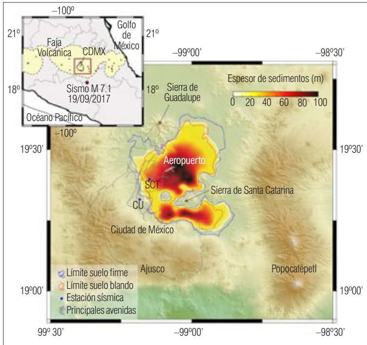
Figura 2. Espesor de la cuenca sedimentaria donde se encuentra gran parte de la Ciudad de México. Nótese la localización del terremoto del 19 de septiembre en el cuadro de la parte superior izquierda. Los puntos azules indican los sitios de dos estaciones sísmicas que registraron los terremotos de 1985 y 2017. La región entre los contornos azul y rojo representa la zona de transición entre el suelo firme y el suelo blando.
