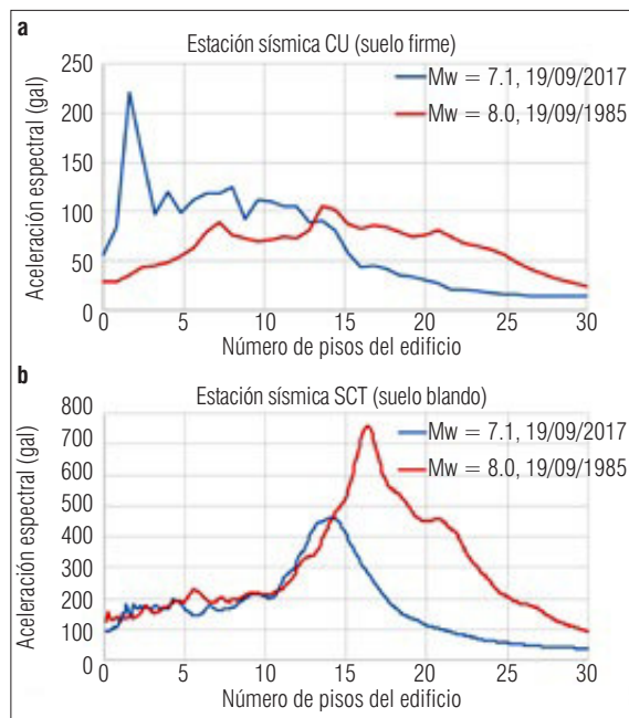
Figura 4. Aceleraciones experimentadas en las azoteas de edificios con diferentes alturas en los sitios CU (a, suelo firme) y SCT (b, suelo blando) (véase figura 2) para los sismos del 19 de septiembre de 1985 (rojo) y de 2017 (azul). 1 gal = 1 cm/s 2 . Las aceleraciones reportadas corresponden al promedio geométrico de ambas componentes horizontales del movimiento.
