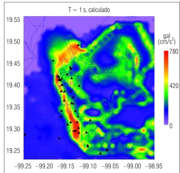
Figura 5. Mapa de aceleraciones espectrales para periodos de 1 segundo, correspondientes a la respuesta de estructuras de 7 a 10 pisos. Los triángulos negros muestran las localizaciones de los edificios colapsados o fuertemente dañados.
