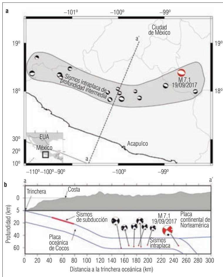
Figura 1. Localizaciones del sismo de magnitud 7.1 del 19 de septiembre de 2017 (color rojo) y de algunos otros del mismo tipo en la región. Las pelotas de playa ilustran la orientación de las fallas y la dirección en que se deslizaron. Todas estas son fallas de tipo normal.
