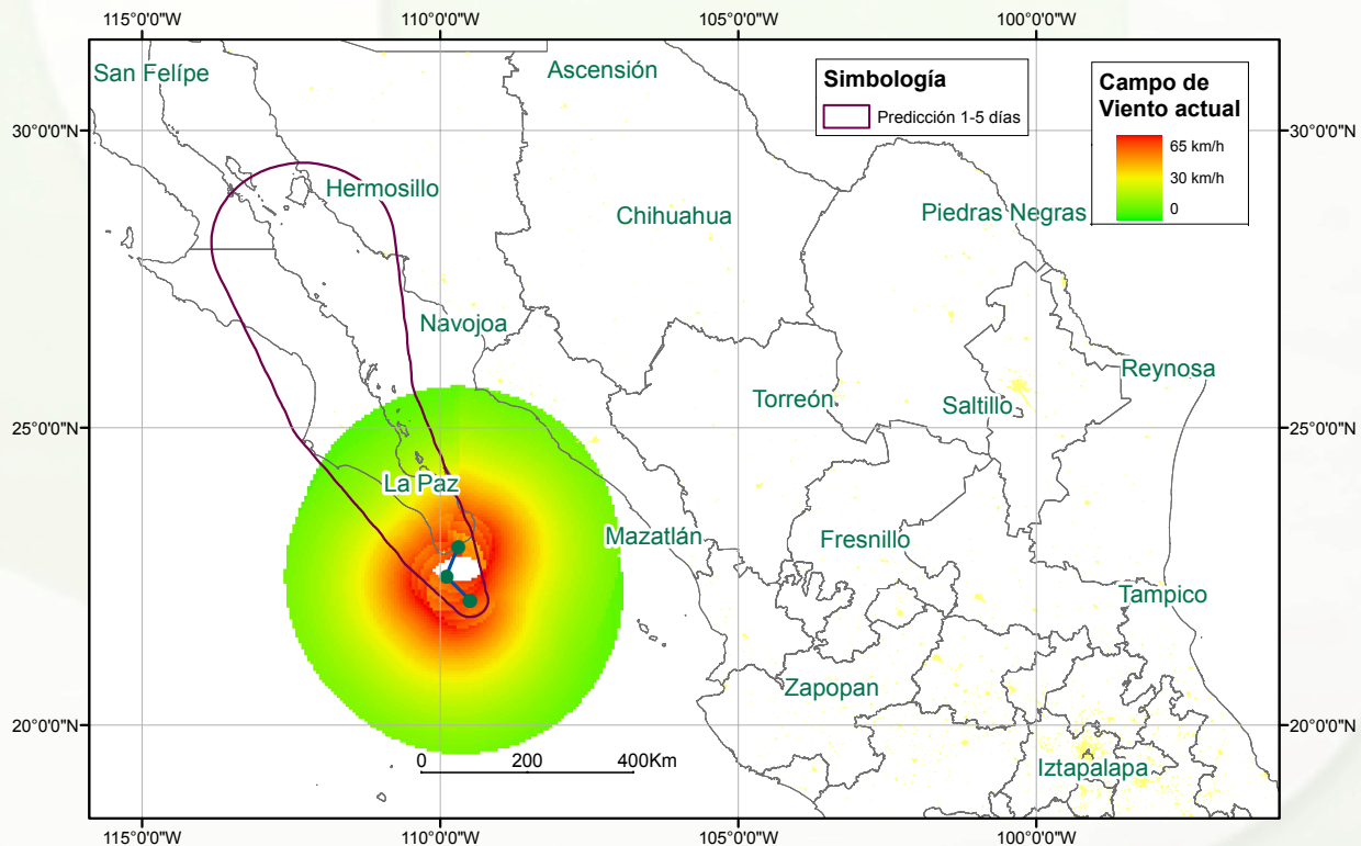
Figura 1. Pronóstico, trayectoria y campos de vientos de la tormenta tropical Georgette. La línea color púrpura representa el pronóstico de la trayectoria para 1 a 5 días. Trayectoria: Unisys Weather, Pronóstico: Centro Nacional de Huracanes y Campos de vientos con modelo ERN.
