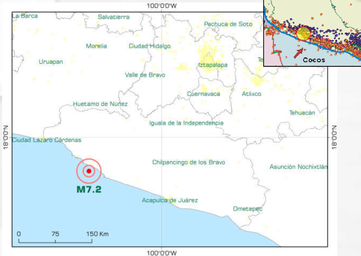
Figura 1. Ubicación del epicentro del sismo de 7.2 del 18 de abril del 2014 con datos del SSN
