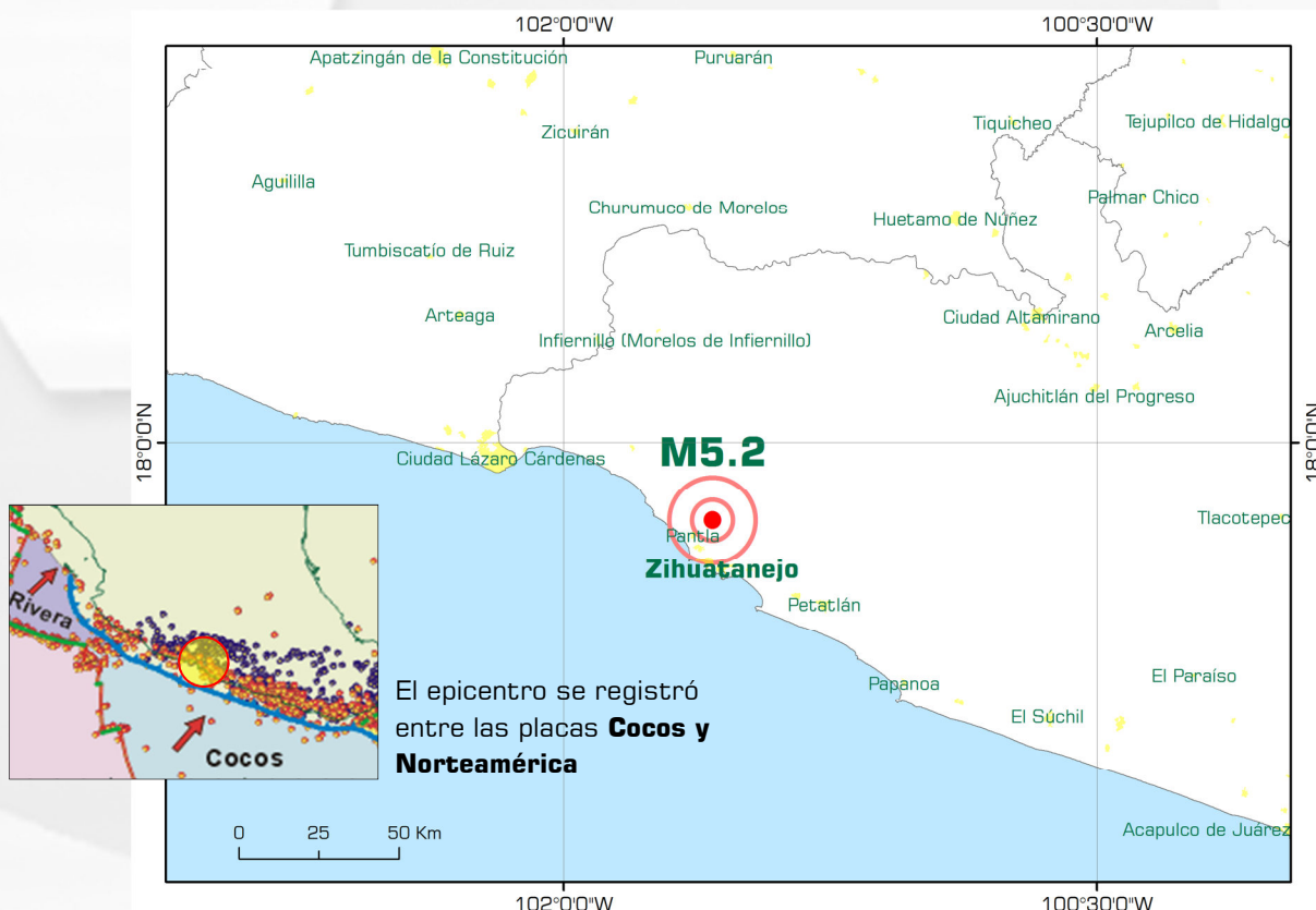
Figura 1. Ubicación del epicentro del sismo de 5.2 del 11 de abril del 2013 de acuerdo al SSN
