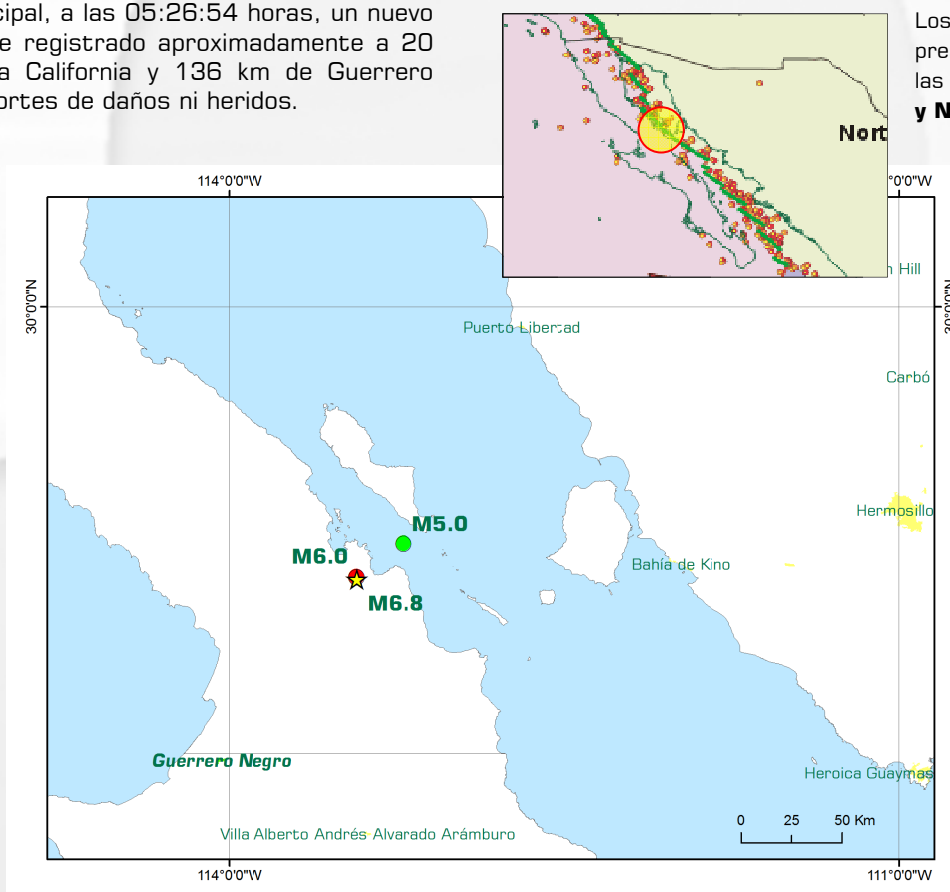
Figura 1. Ubicación de los tres sismos que se presentaron en Baja California en las primeras horas del día 12 de abril. El sismo más intenso es el que se representa con la estrella amarilla, de magnitud 6.8
